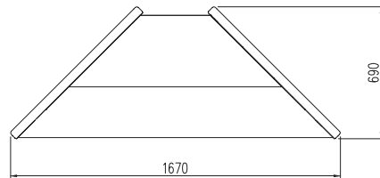
Detalle mueble caja (frente) Cash counter (front view)
